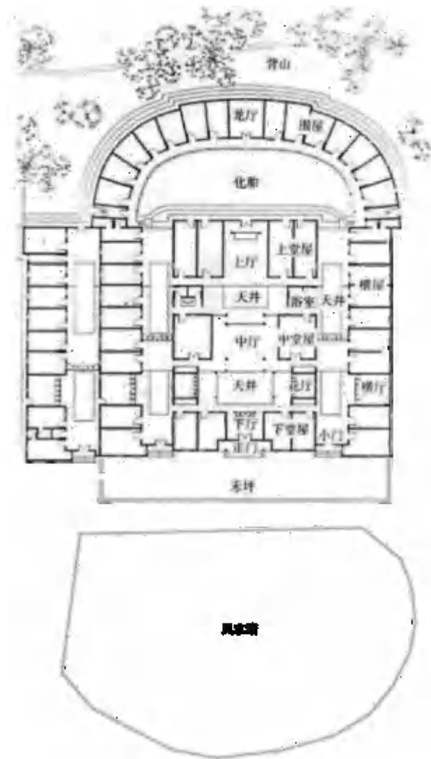
安善庐 平面形制图
